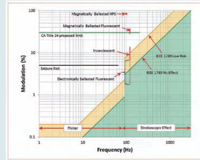
图: 低风险和不可察觉到的影响水平的闪烁频率和波动深度函数关系文件对无频闪判定准则为:
